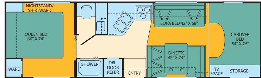
OPT. 026 20' AWNING
