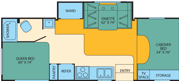
OPT. 026 17' AWNING
